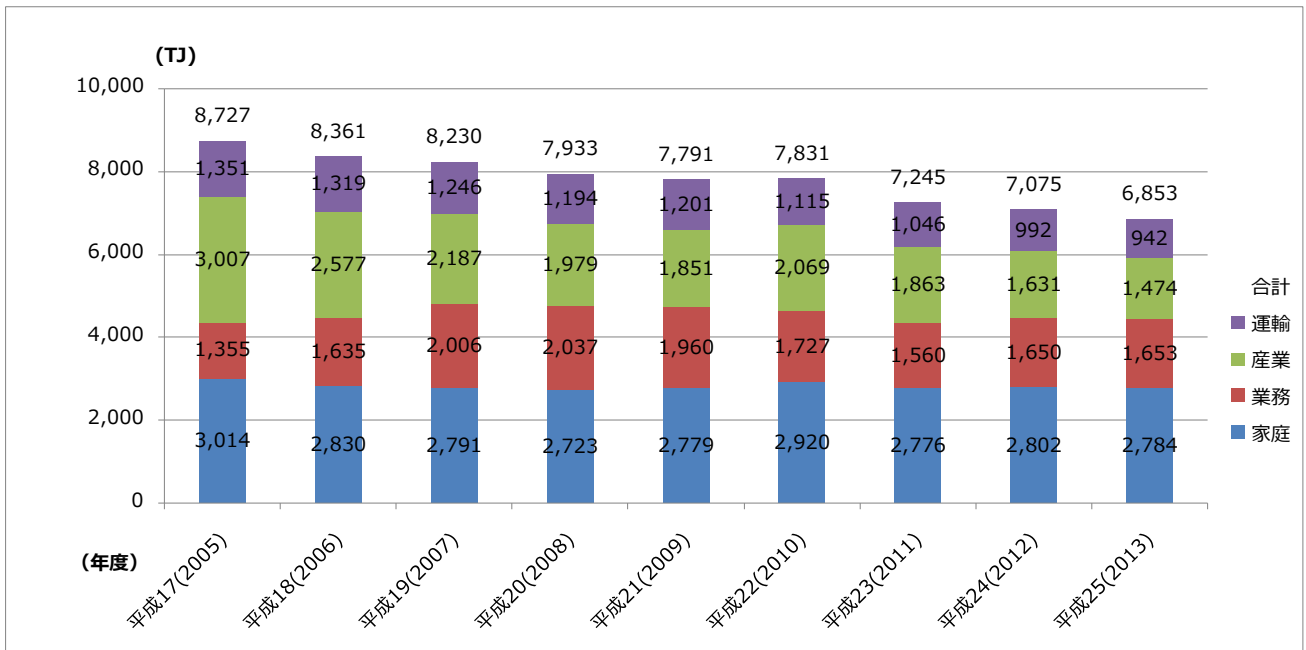
図 2 小平市の部門別エネルギー消費量の推移
