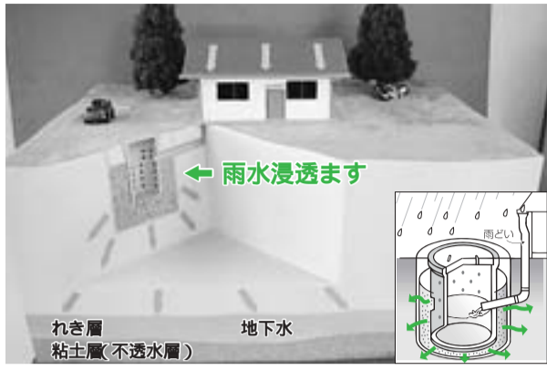
雨水浸透ますの模型
