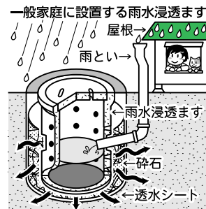
一般家庭に設置する雨水浸透ます
